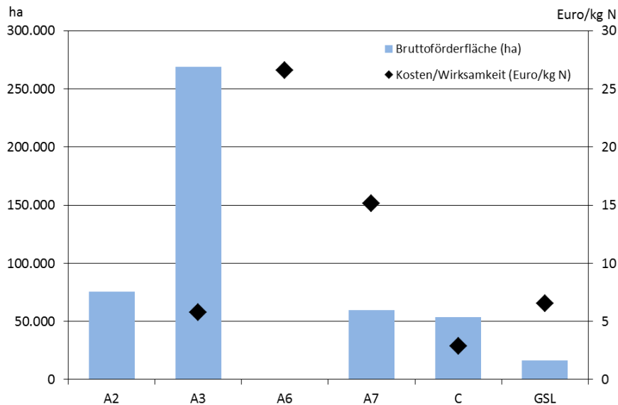
Abbildung 13: Kosten-Wirksamkeitsrelationen der Agrarumweltmaßnahmen mit Wasserschutzzielen bezogen auf den Indikator ‚Minderung von N-Bilanzen‘
